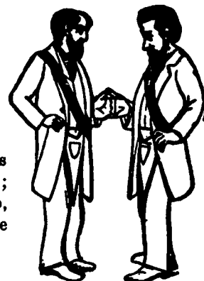
Token
