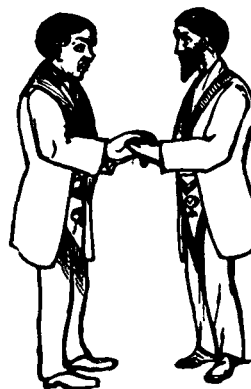
Token.
