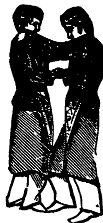
Token
