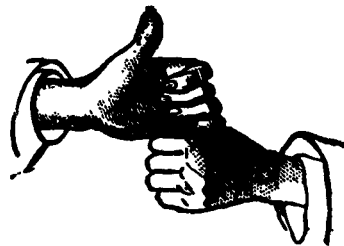
Token
