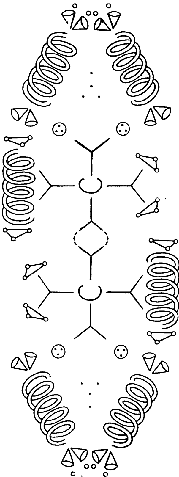
FIG. 200. TARTARIC ACID
