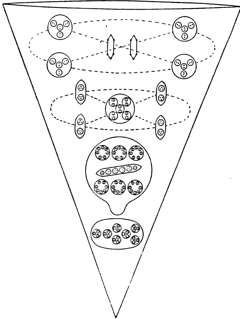
FIG. 79. YTTRIUM
