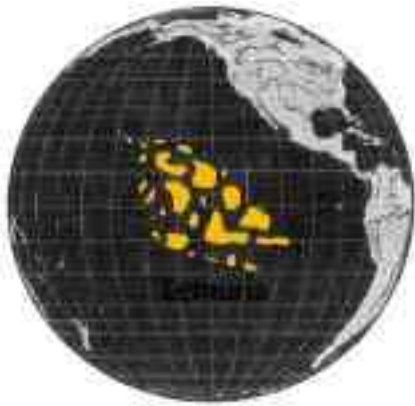
Fig. 3-12. Lemuria.
