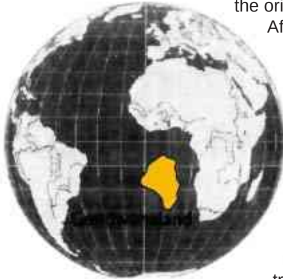
Fig. 3-11. Gondwanaland
